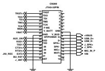
J-TAG 32 PINS
