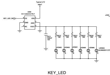
KEY_LED
